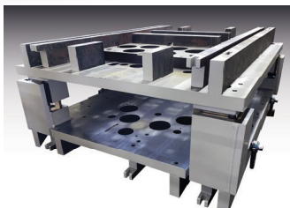
PORTA-TROQUELES DE TALÓN
