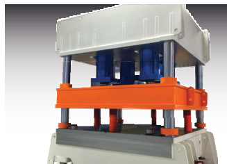
TROQUELES MULTI-PLACA
